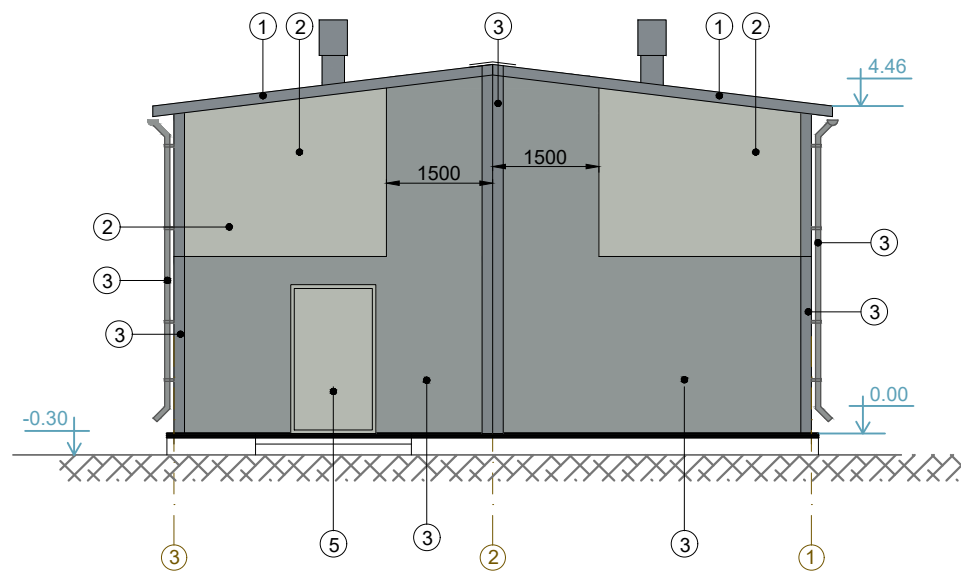
Fasāde asīs 2-1 M 1:100
