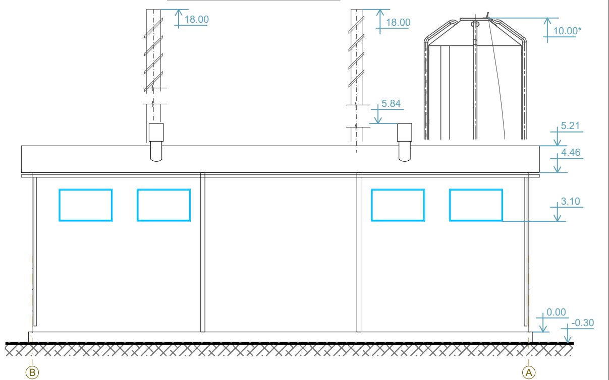
Fasāde asis B-A M 1:100
