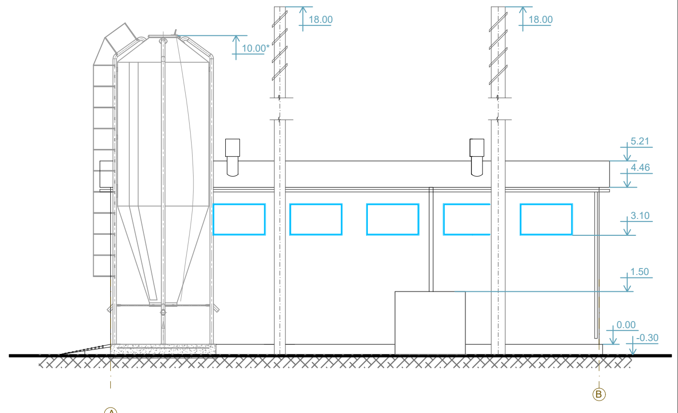
Fasāde asis B-A M 1:100
